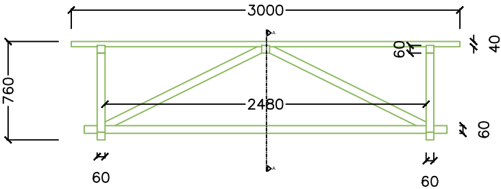
ALZADO ELEVATION
