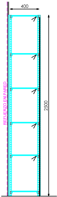
SECCION BALDAS
