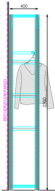
ALZADO LATERAL
