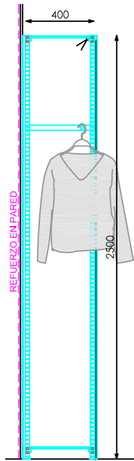
SECCION BARRA H190
