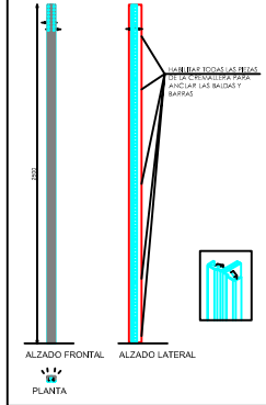
BALDA EXTRAIBLE MODULO 100
