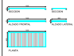
BARRA EXTRAIBLE MODULO 100
