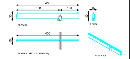
DETALLE FRONTALES EXTRAIBLES
