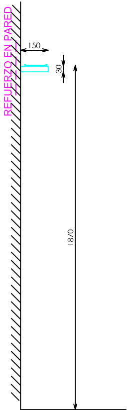
SECCION
