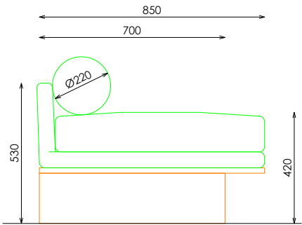
ALZADO LATERAL
