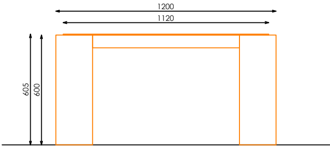
ALZADO FRONTAL
