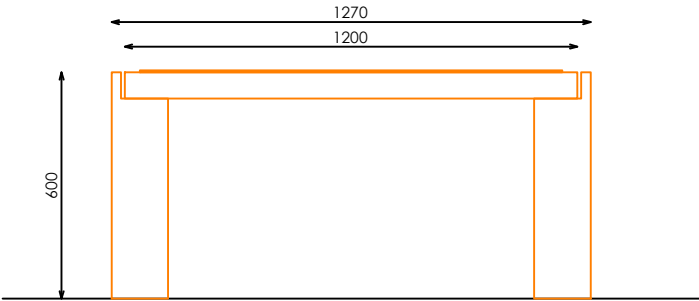
ALZADO LATERAL
