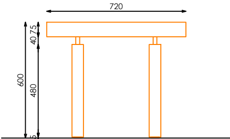
ALZADO LATERAL
