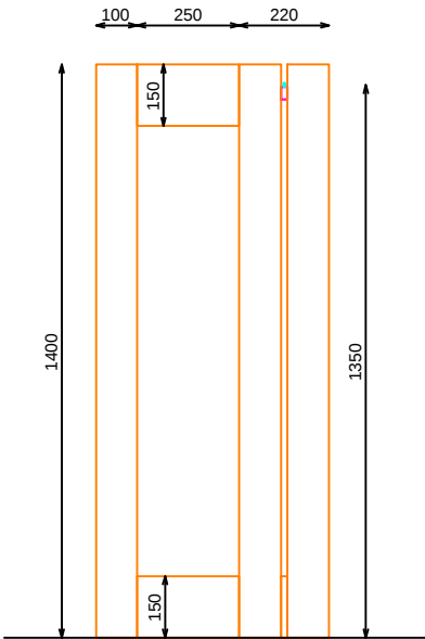
ALZADO IZQUIERDO
