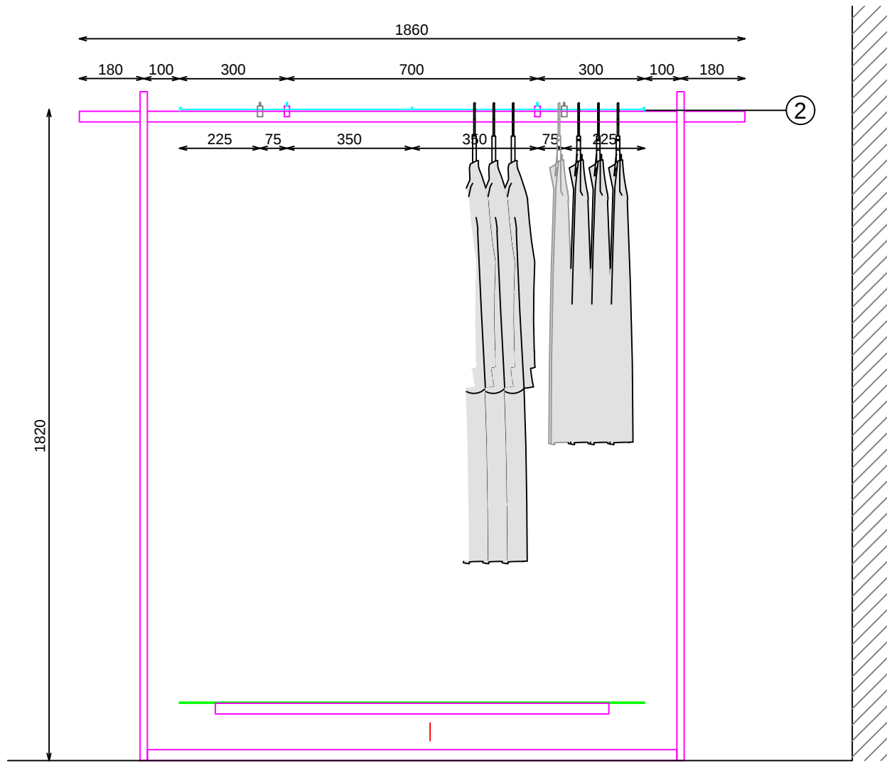
ALZADO FRONTAL
