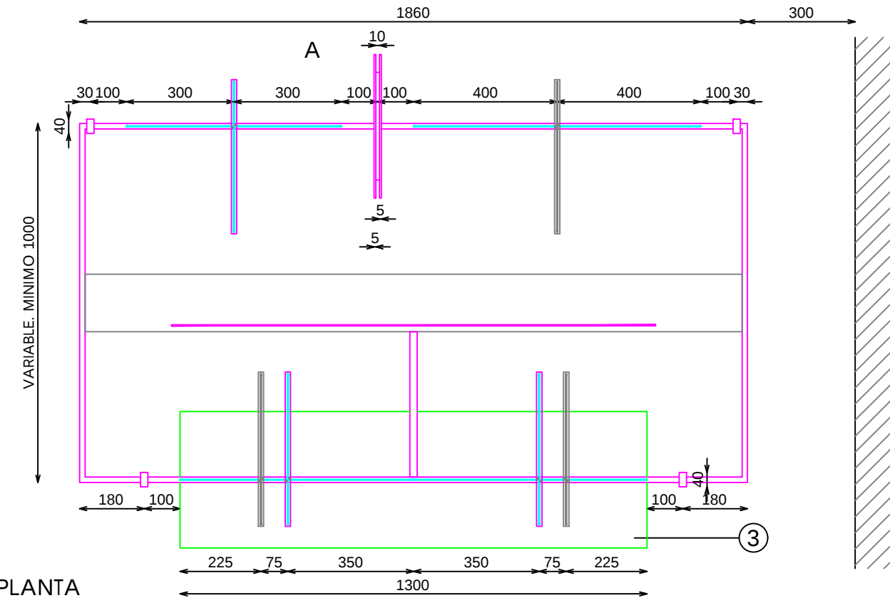
PLANTA
