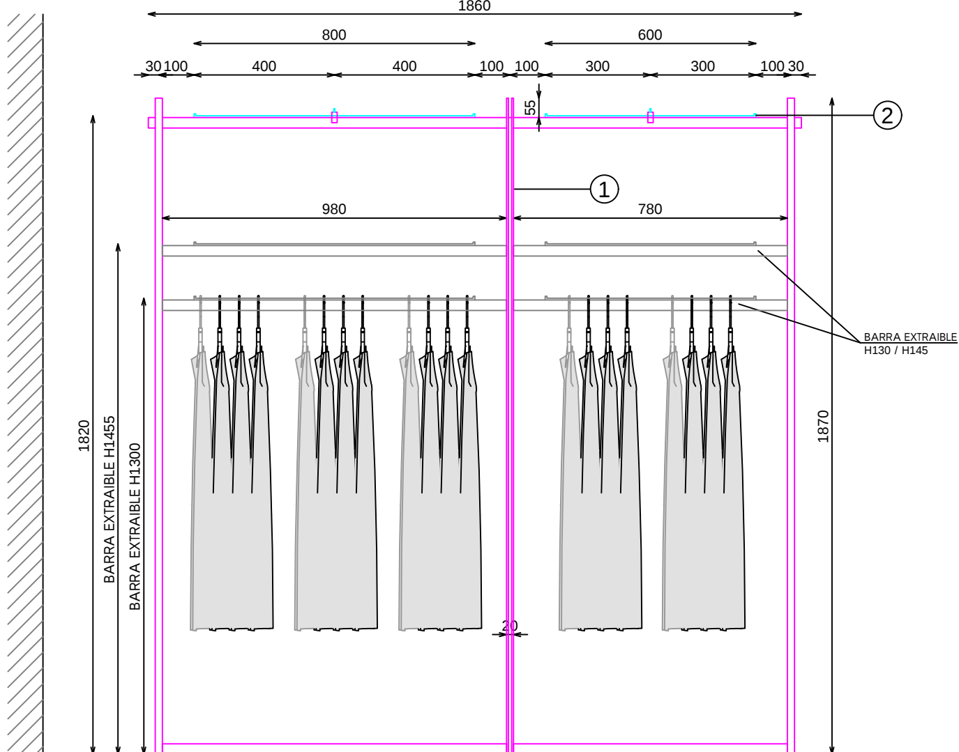
ALZADO TRASERO
