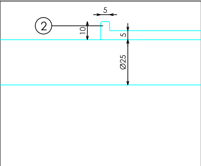
DETALLE ANTIROCE
