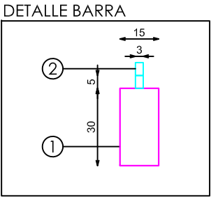
DETALLE BARRA
