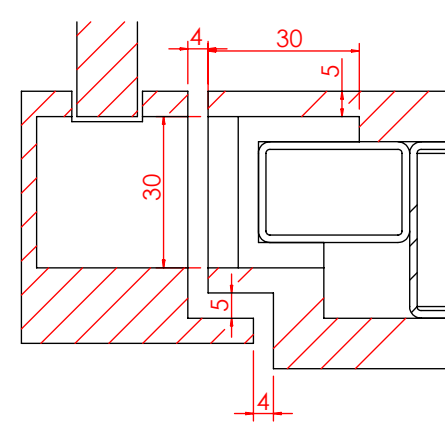
局部视图 AI 比例 2 : 3
