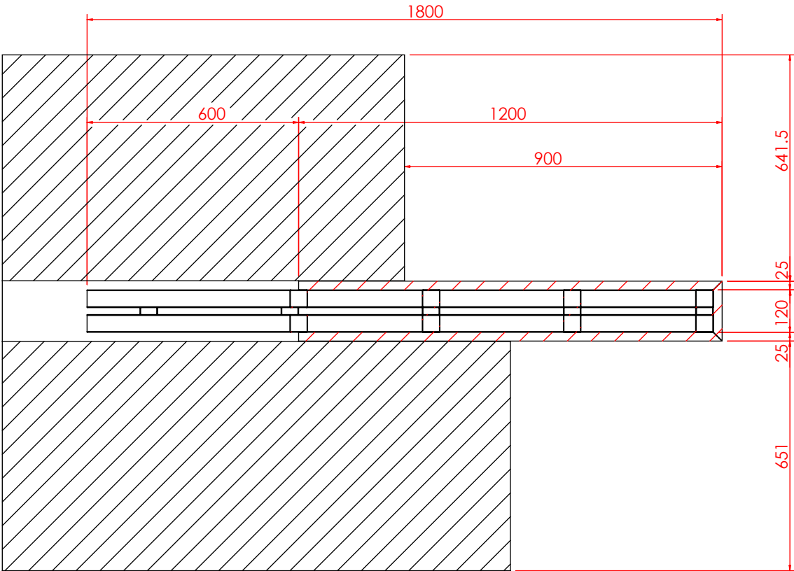
剖面 AG-AG 比例 1 : 15
