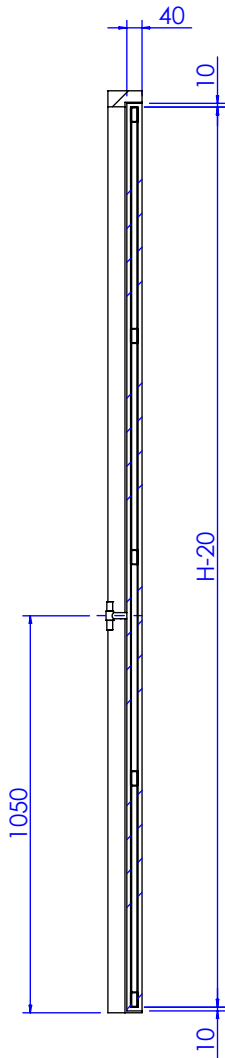
剖面 AI-AI
