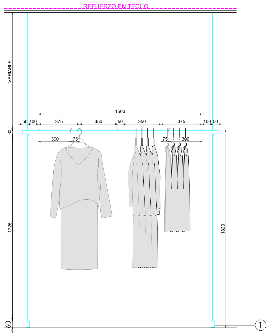
ALZADO FRONTAL
