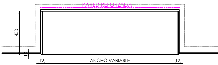
PLANTA
