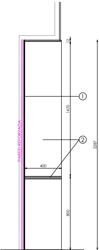
SECCIÓN
