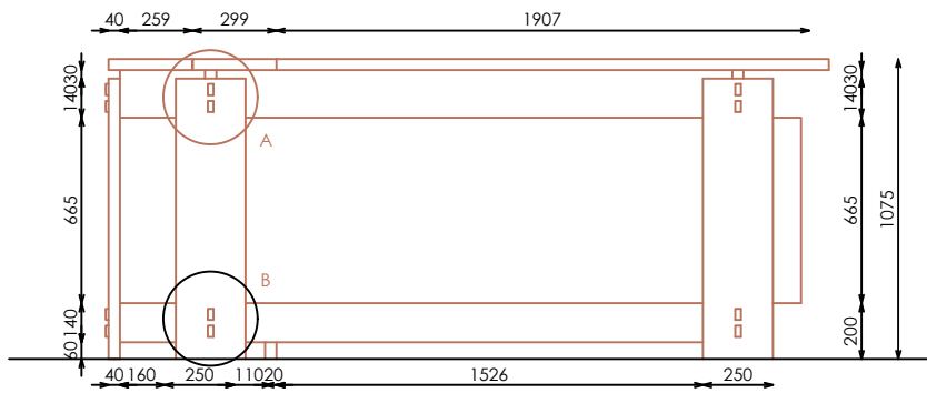
ALZADO DERECHO
