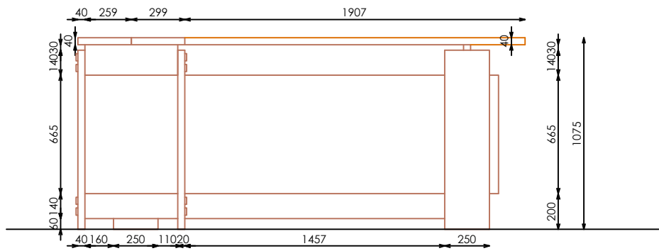
ALZADO TRASERO
