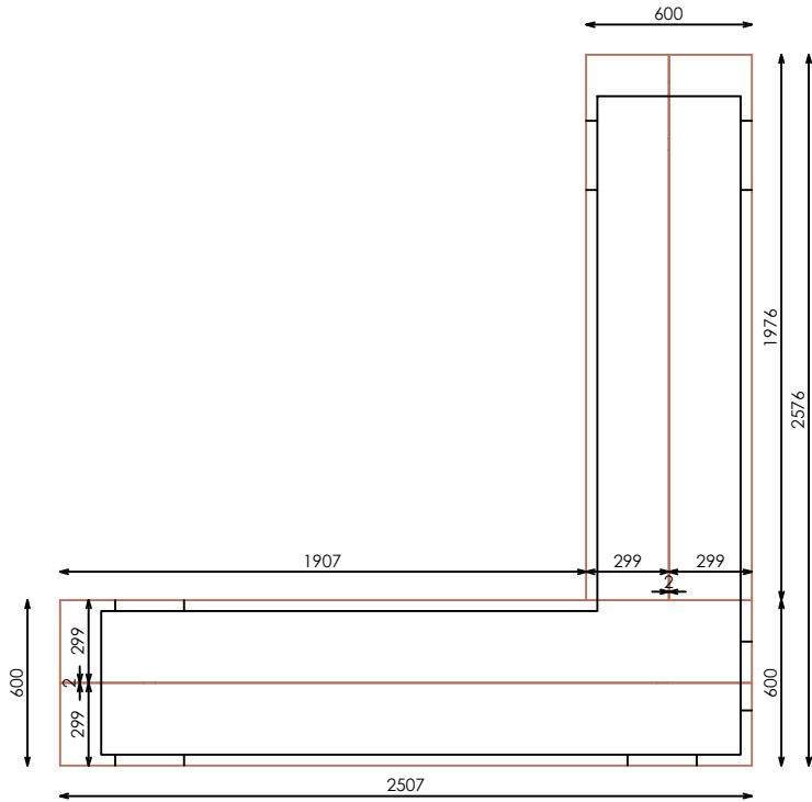
PLANTA
