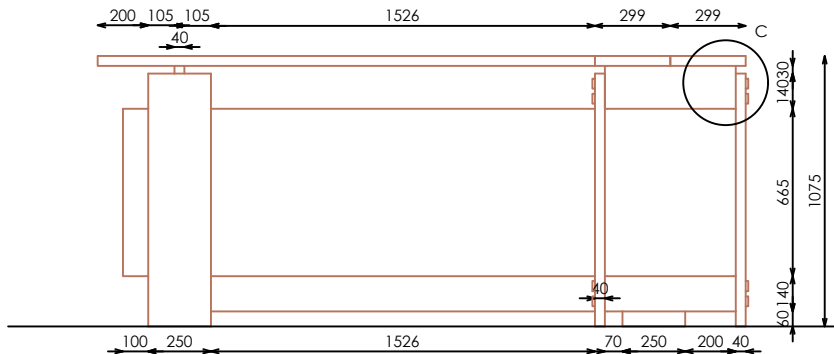
ALZADO IZQUIERDO
