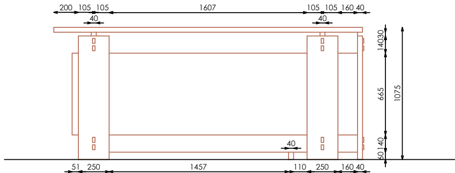
ALZADO FRONTAL
