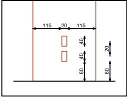
DETALLE C
