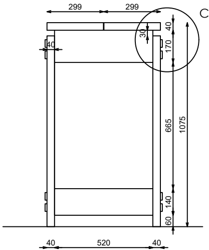
ALZADO LATERAL
