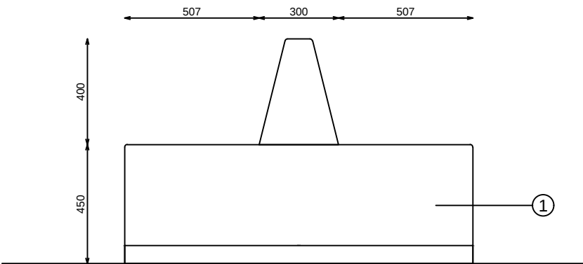
ALZADO LATERAL
