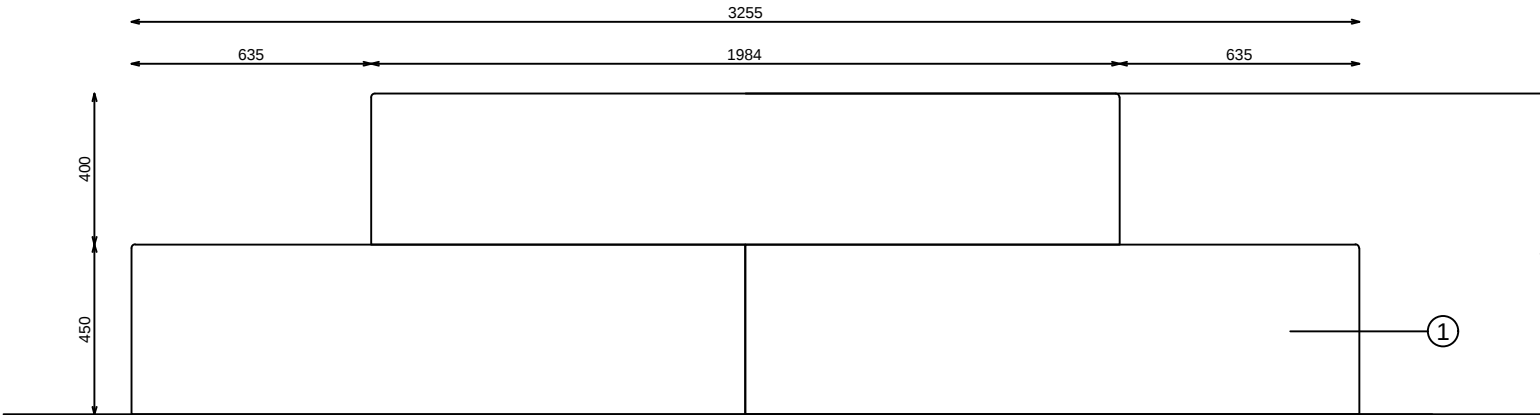
ALZADO FRONTAL
