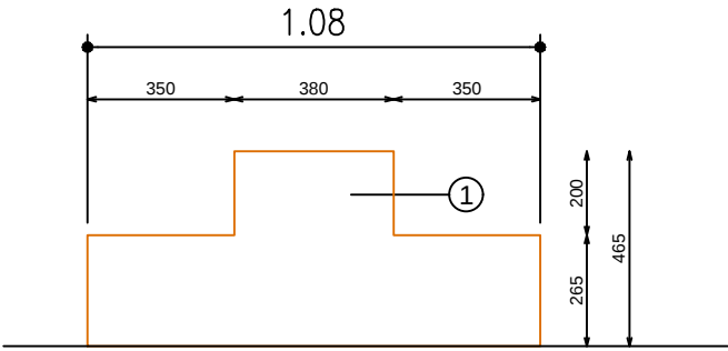
PERFIL
