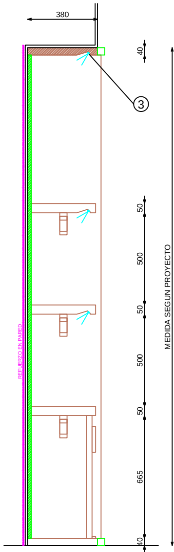
SECCIÓN BALDAS
