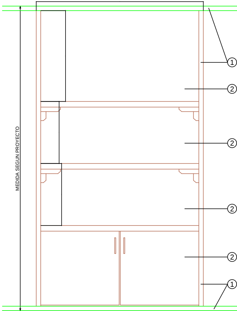
ALZADO
