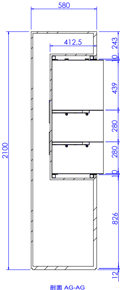
剖面 AG-AG
