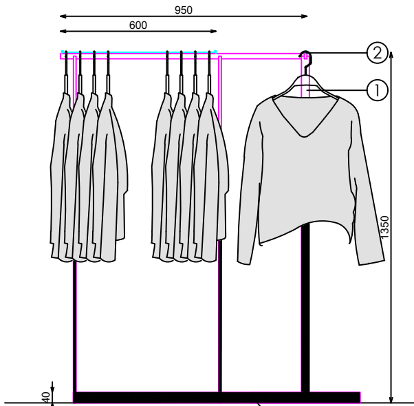
ALZADO LATERAL
