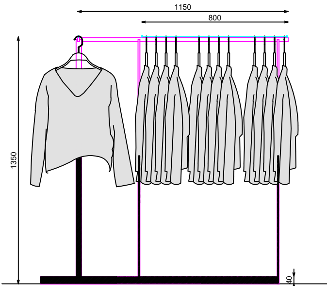
ALZADO FRONTAL
