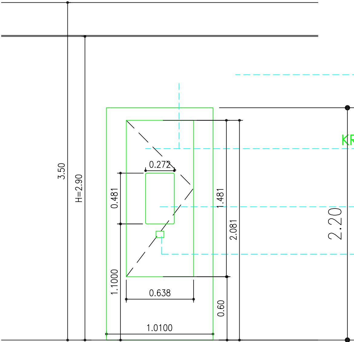
ALZADO
