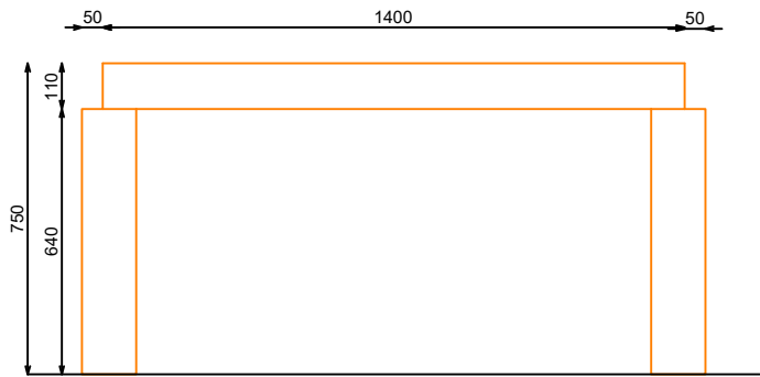
ALZADO FRONTAL
