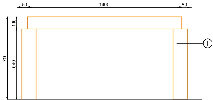
ALZADO LATERAL
