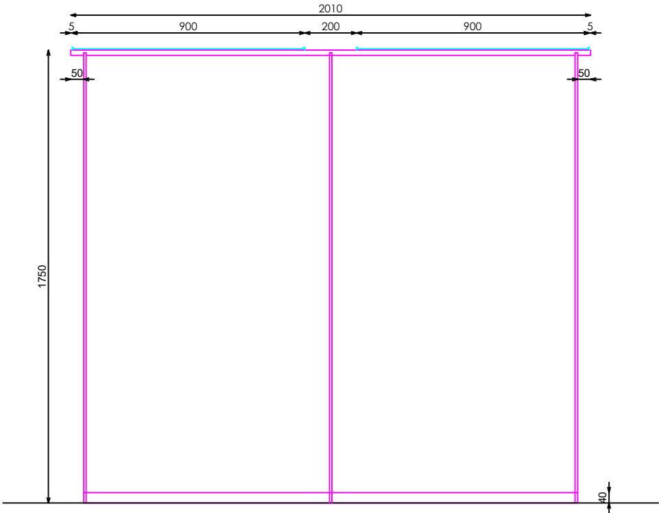
ALZADO
