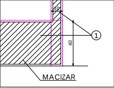
DETALLE C
