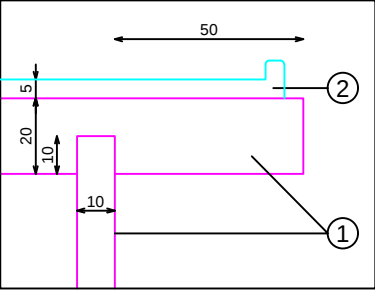
DETALLE B
