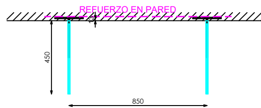
PLANTA
