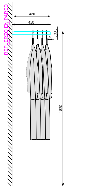
SECCION
