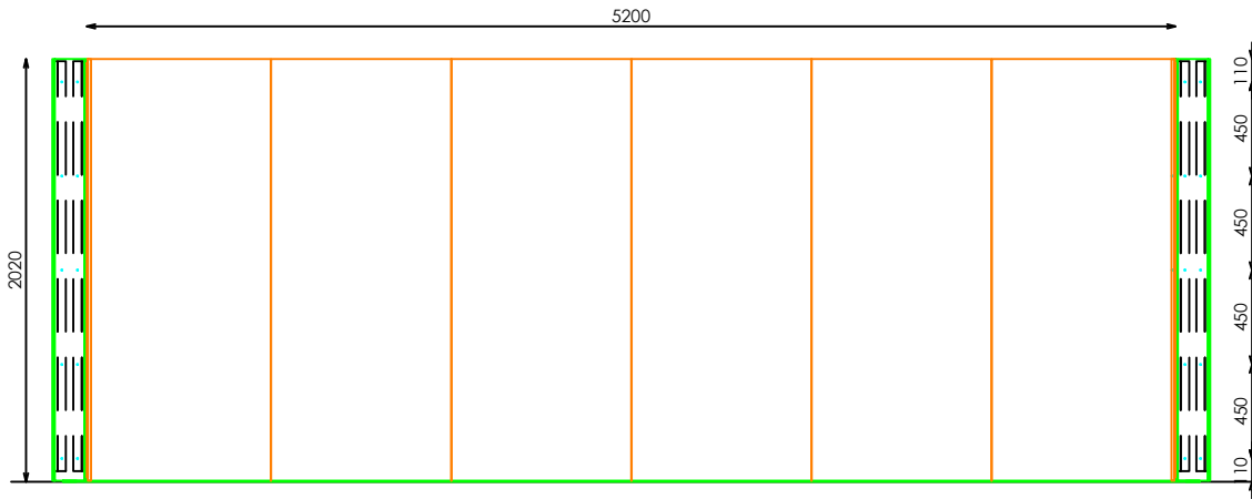
ALZADO FRONTAL
