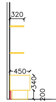
PERFIL SIDE ELEVATION
