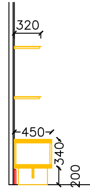
SECCIÓN AA SECTION AA
