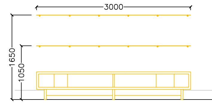
ALZADO ELEVATION
