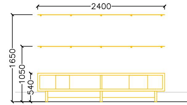
ALZADO ELEVATION
