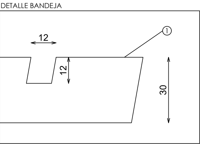
DETALLE BANDEJA
