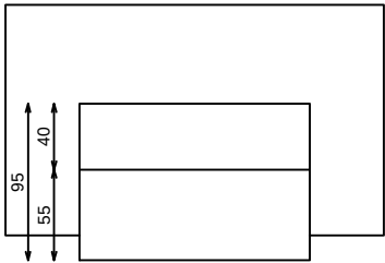
PERFIL DCHO
