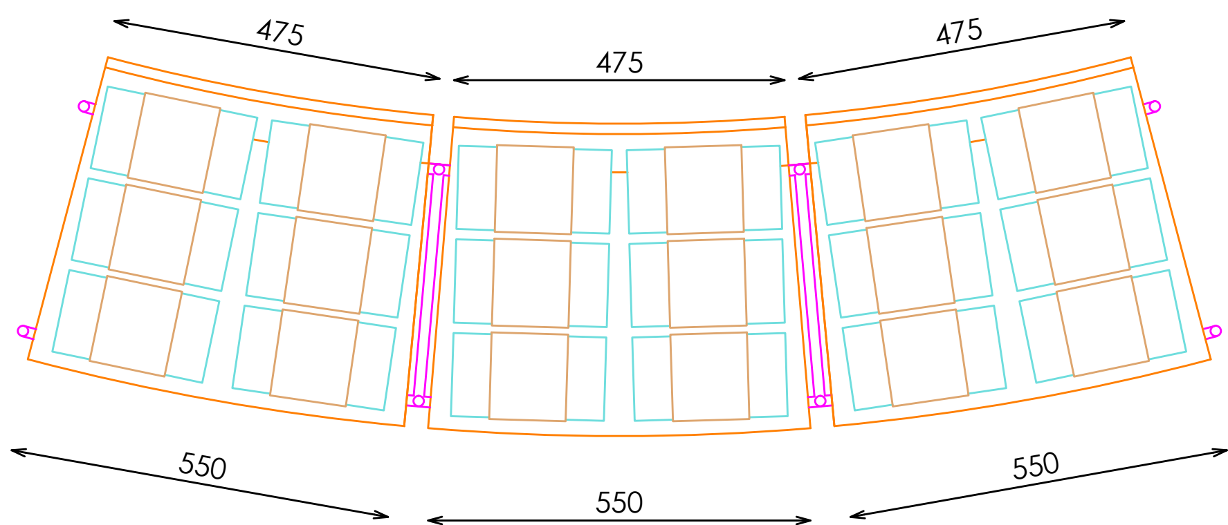
PLANTA
