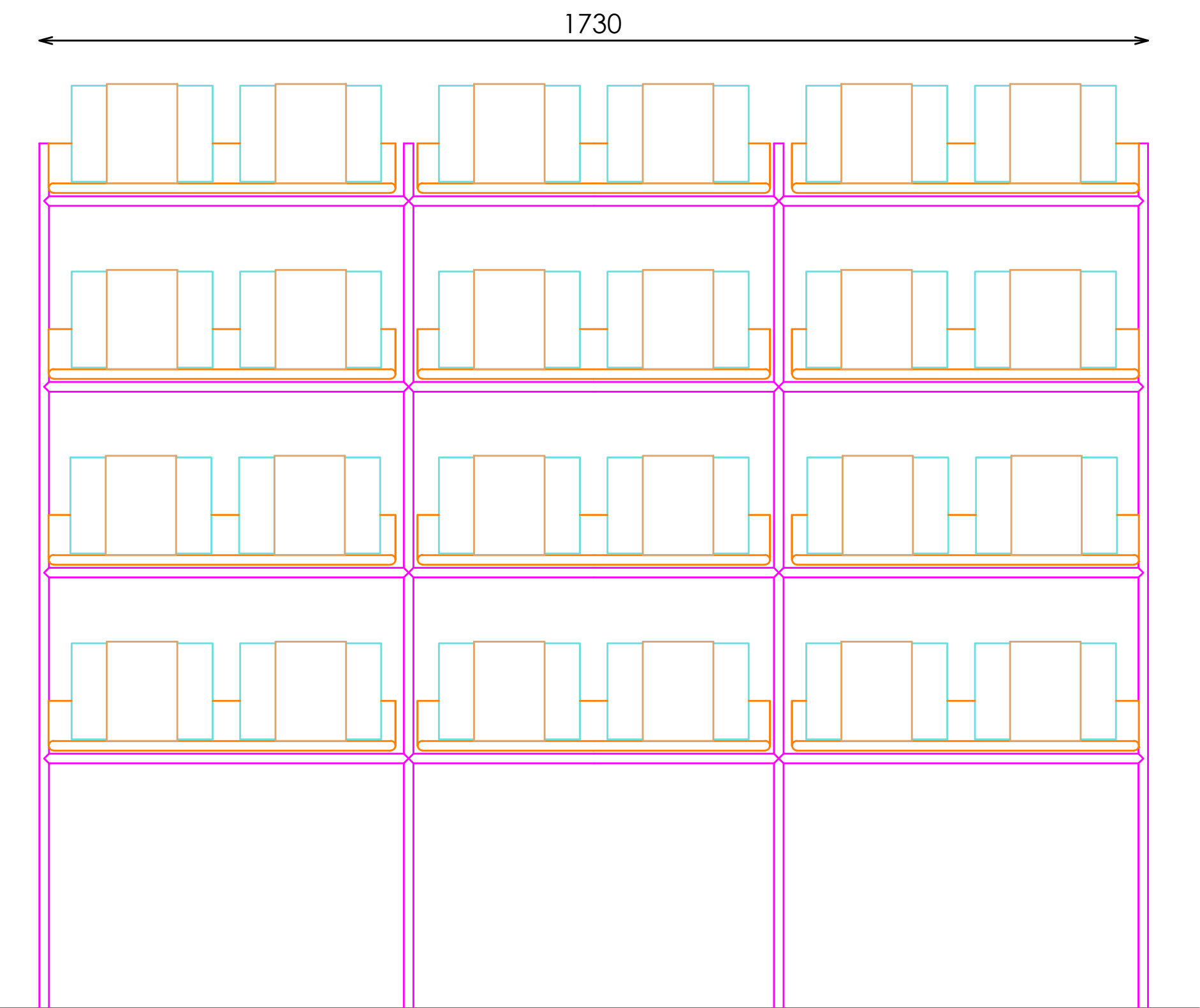
ALZADO FRONTAL
