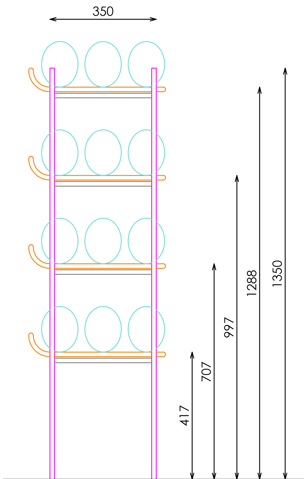
ALZADO LATERAL
