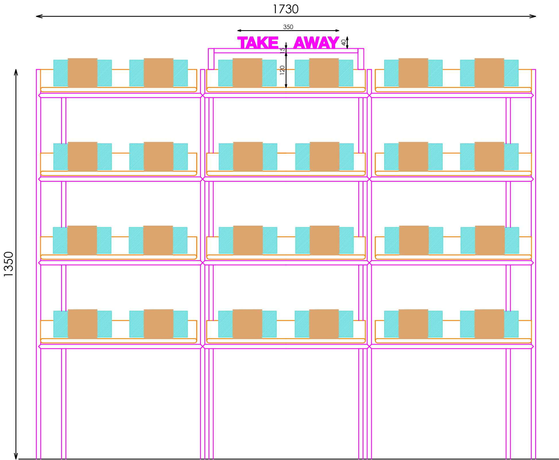
ALZADO FRONTAL
