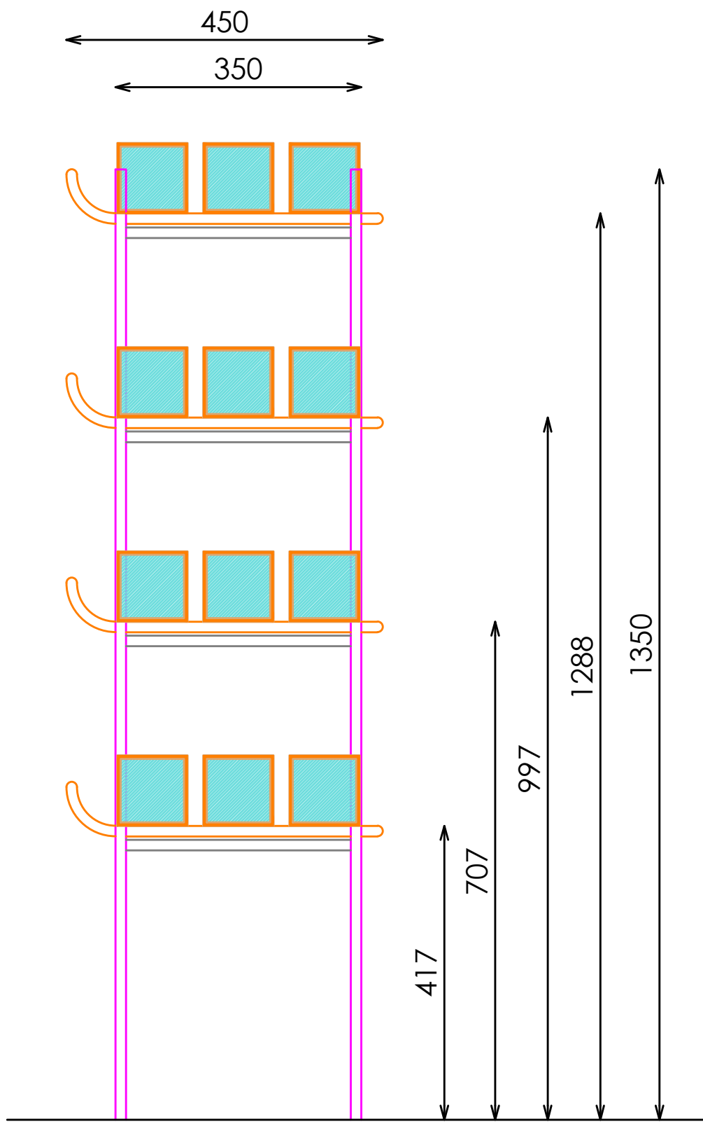
ALZADO LATERAL
