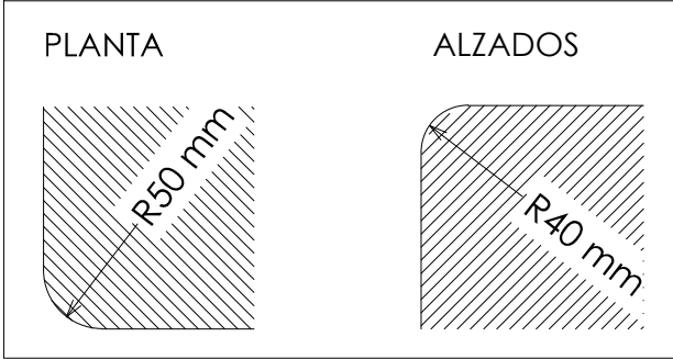
DETALLE CURVATURAS
