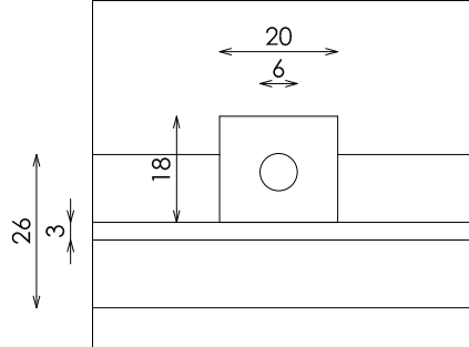
DETALLE BARRA ANCLAJE FROTANLES
