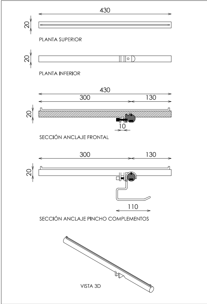
DETALLE ANCLAJE FRONTALES EXTRAIBLES
