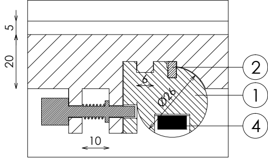
DETALLE ILUMINACION TARIMA
