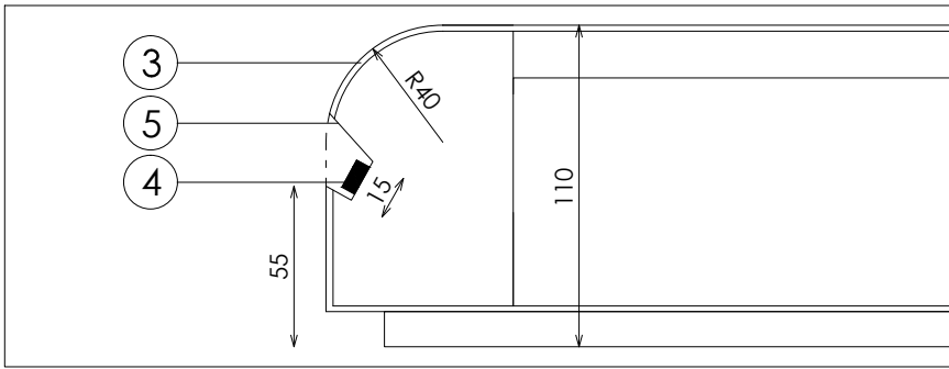
DETALLE ILUMINACION TARIMA
