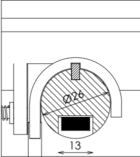
DETALLE ANCLAJE PINCHO COMP.
