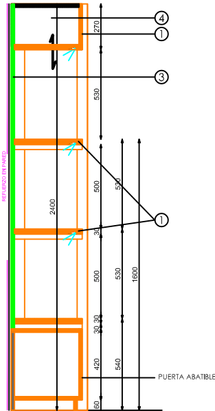
SECCION
