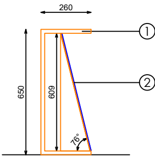
SECCIÓN
