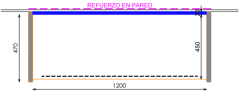
PLANTA SECCIONADA
