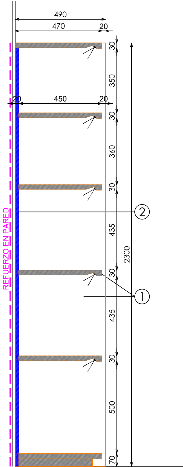
SECCION
