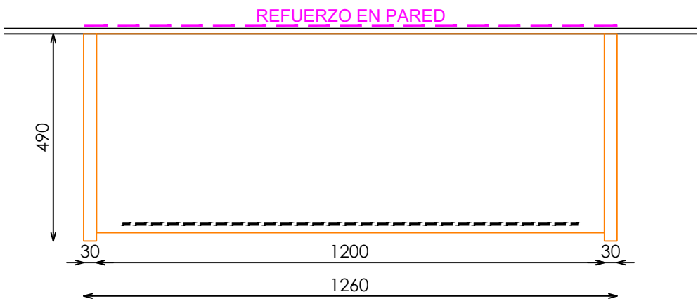
PLANTA
