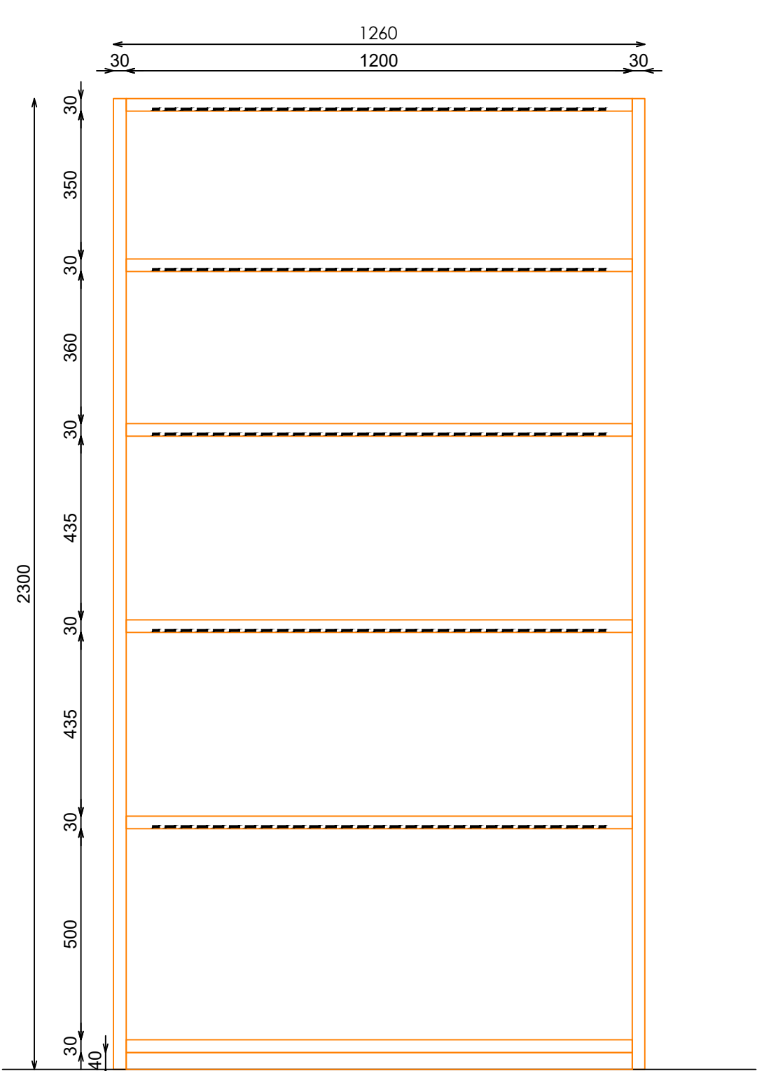
ALZADO
