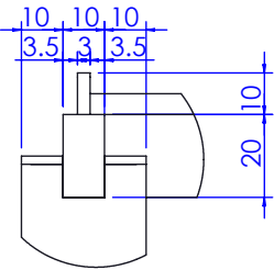
局部视图 AN 比例 1 : 2
