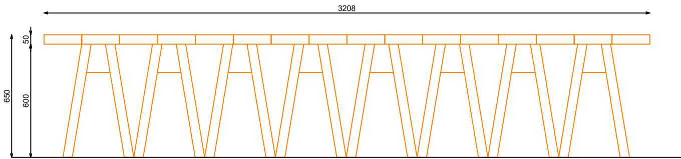
ALZADO
