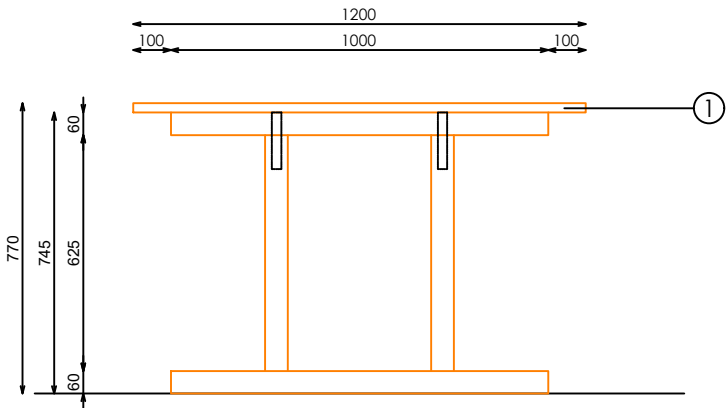
ALZADO LATERAL
