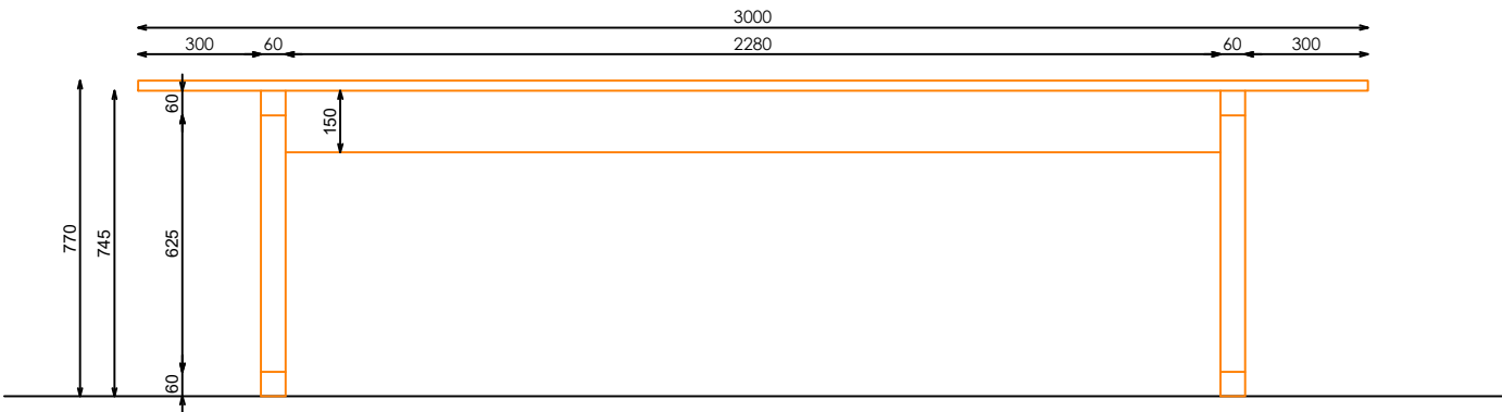
ALZADO FRONTAL
