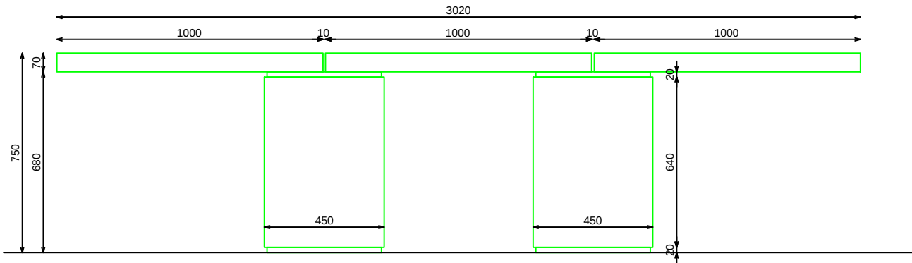
ALZADO FRONTAL
