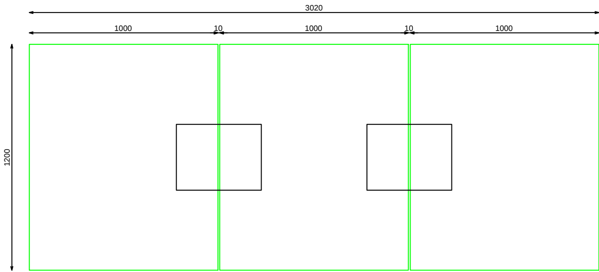
PLANTA
