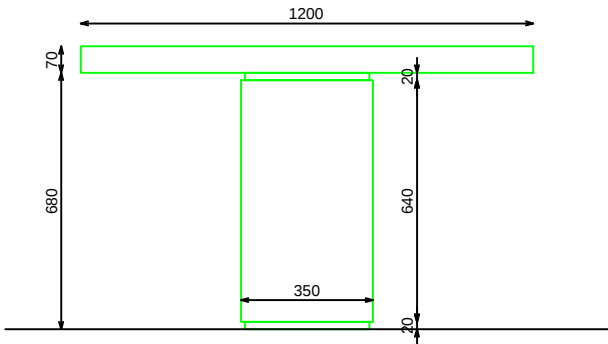
ALZADO LATERAL
