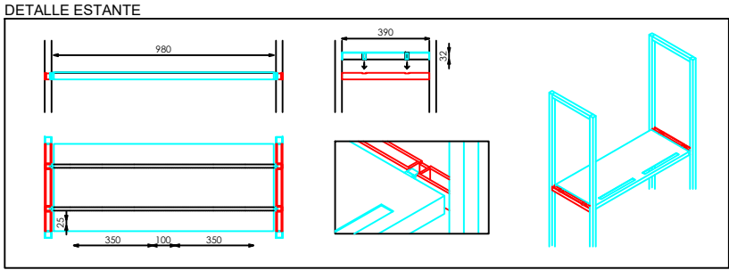
DETALLE ESTANTE
