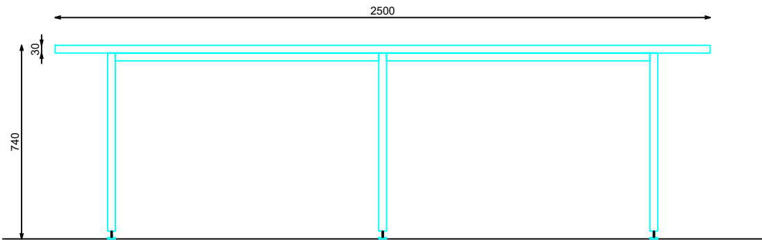
ALZADO FRONTAL
