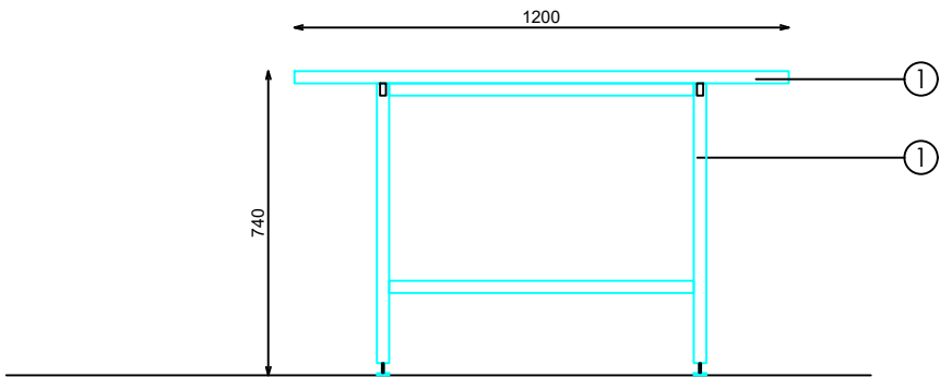
ALZADO LATERAL
