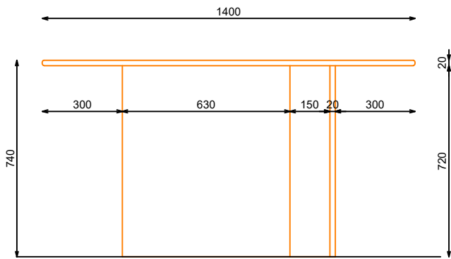
ALZADO FRONTAL
