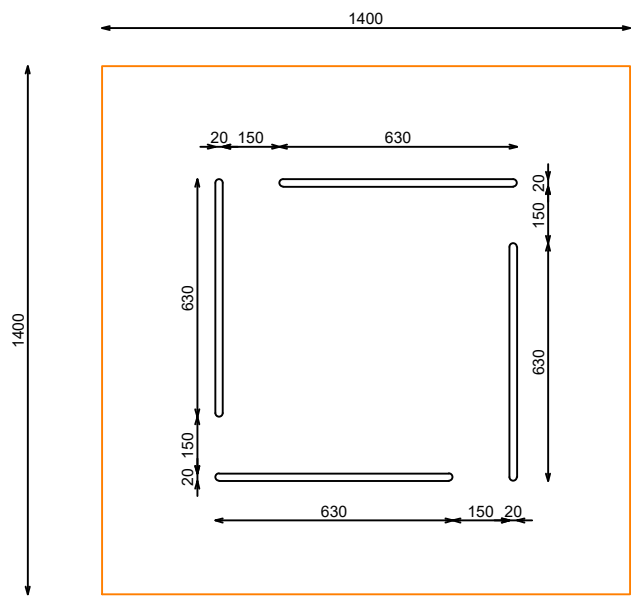
PLANTA
