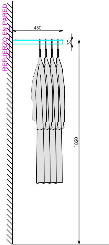
SECCION
