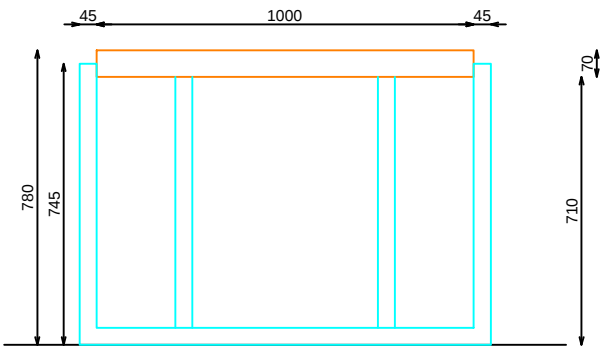
ALZADO LATERAL
