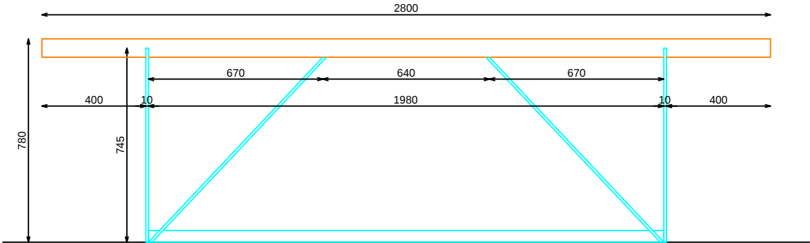
ALZADO FRONTAL
