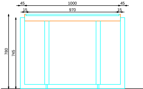
SECCION
