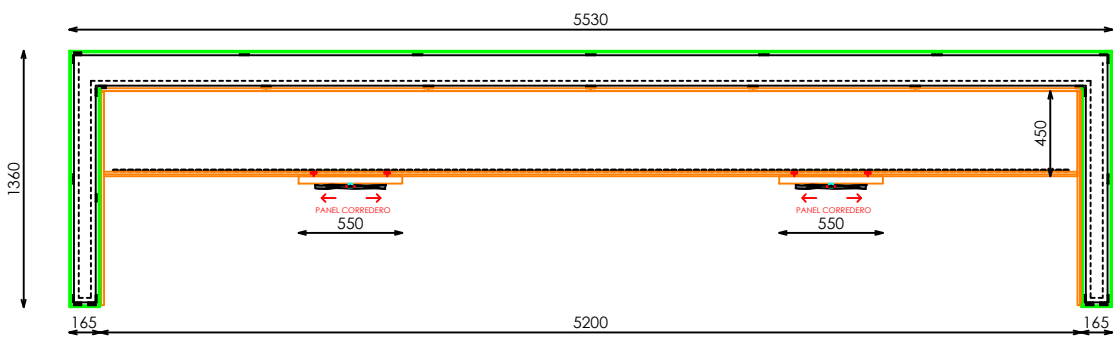
PLANTA
