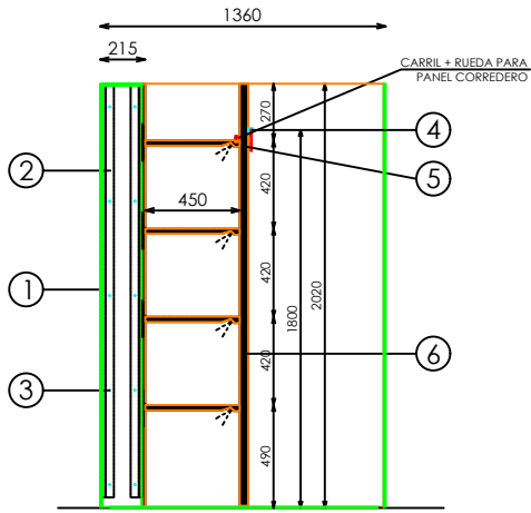
SECCION
