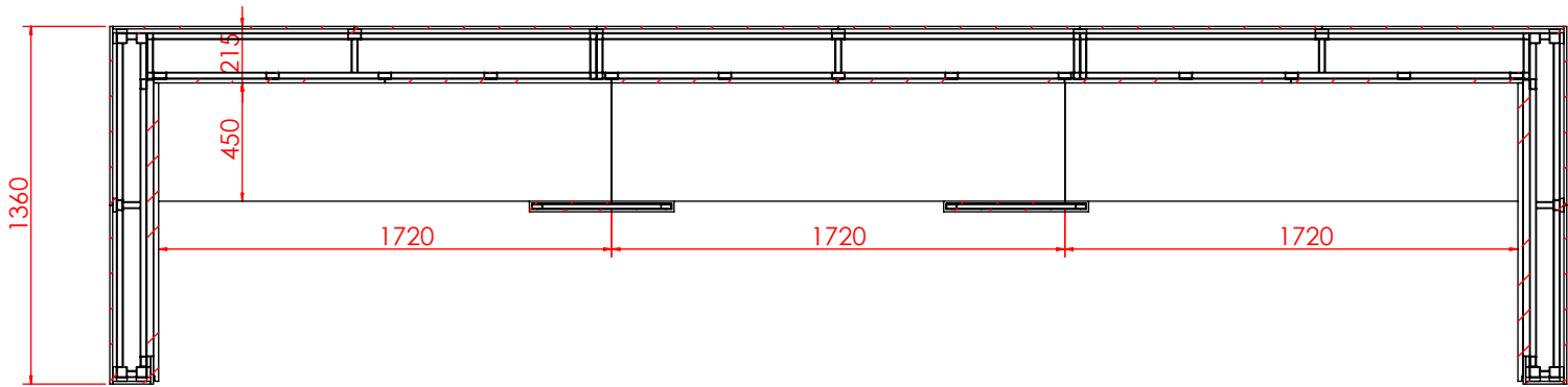
剖面 AJ-AJ
