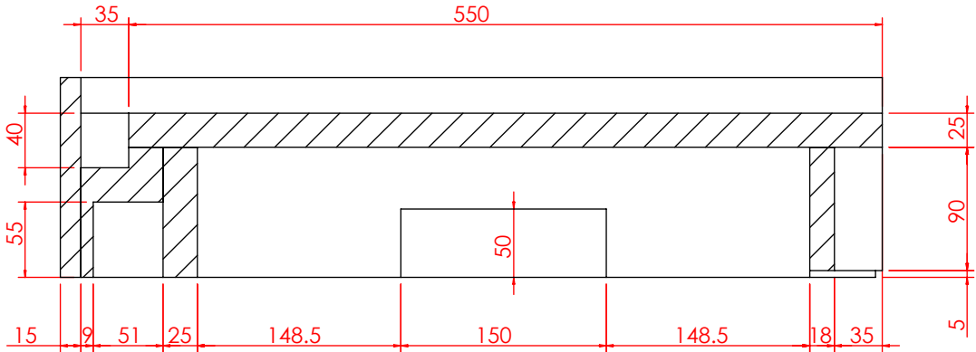
局部视图 AH 比例 1 : 5
