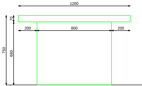
ALZADO FRONTAL
