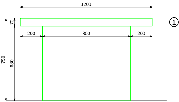
ALZADO LATERAL
