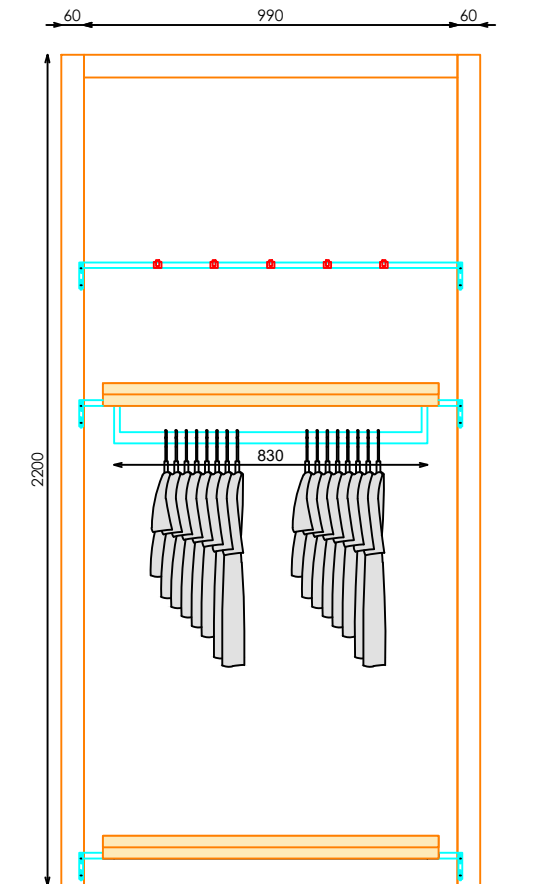
ALZADO
